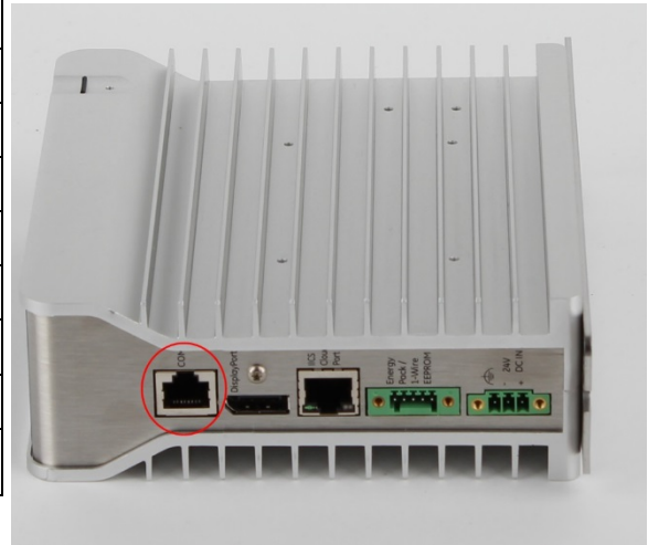
Figure 37: COM1 Port CPE400
